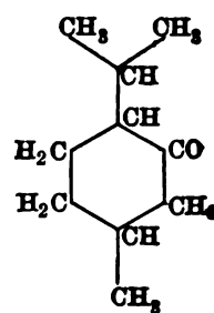
Menthone.
